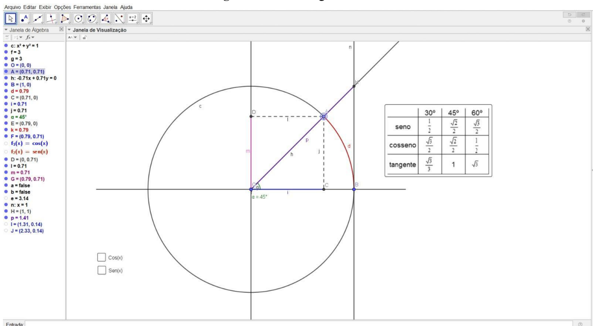
Figura 1 – Ciclo Trigonométrico
