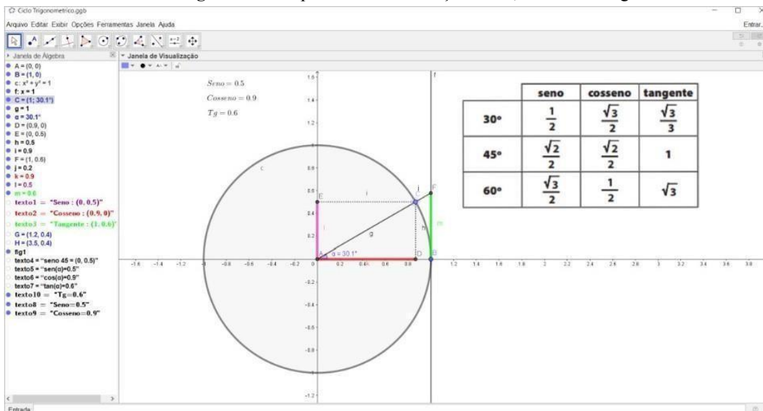
Figura 2 – Comportamento das funções seno, cosseno e tangente
